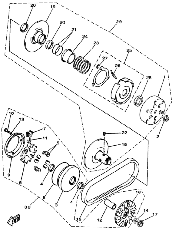
32 CLUTCH
